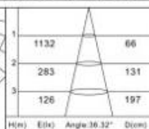
H(m) E(lx) Angle: 36.32° D(cm)
