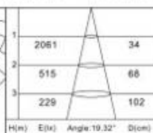
H(m) E(lx) Angle: 19.32° D(cm)
