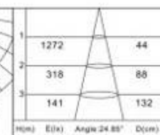
H(m) E(lx) Angle: 24.85° D(cm)
