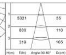
H(m) E(lx) Angle: 30.80° D(cm)
