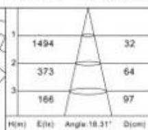
H(m) E(lx) Angle: 18.31° D(cm)
