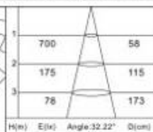
H(m) E(lx) Angle: 32.22° D(cm)
