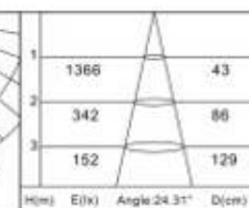
H(m) E(lx) Angle: 24.31° D(cm)
