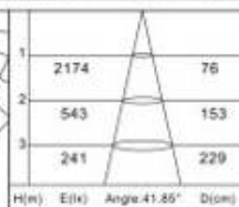
H(m) E(lx) Angle: 41.85° D(cm)
